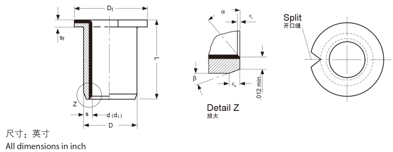
翻边套型号标注方式 Flange Bushing Symbol
